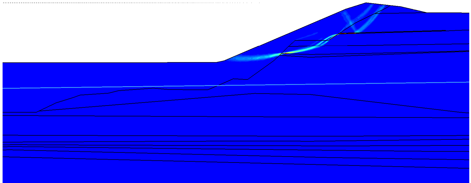
Abbildung 3: Potentieller Versagensmechanismus im prognostischen Zustand mit geplanten Maßnahmen aus Deponieerrichtung
