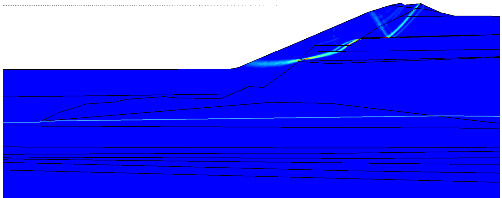
Abbildung 1: Potentieller Versagensmechanismus im aktuellen Zustand
