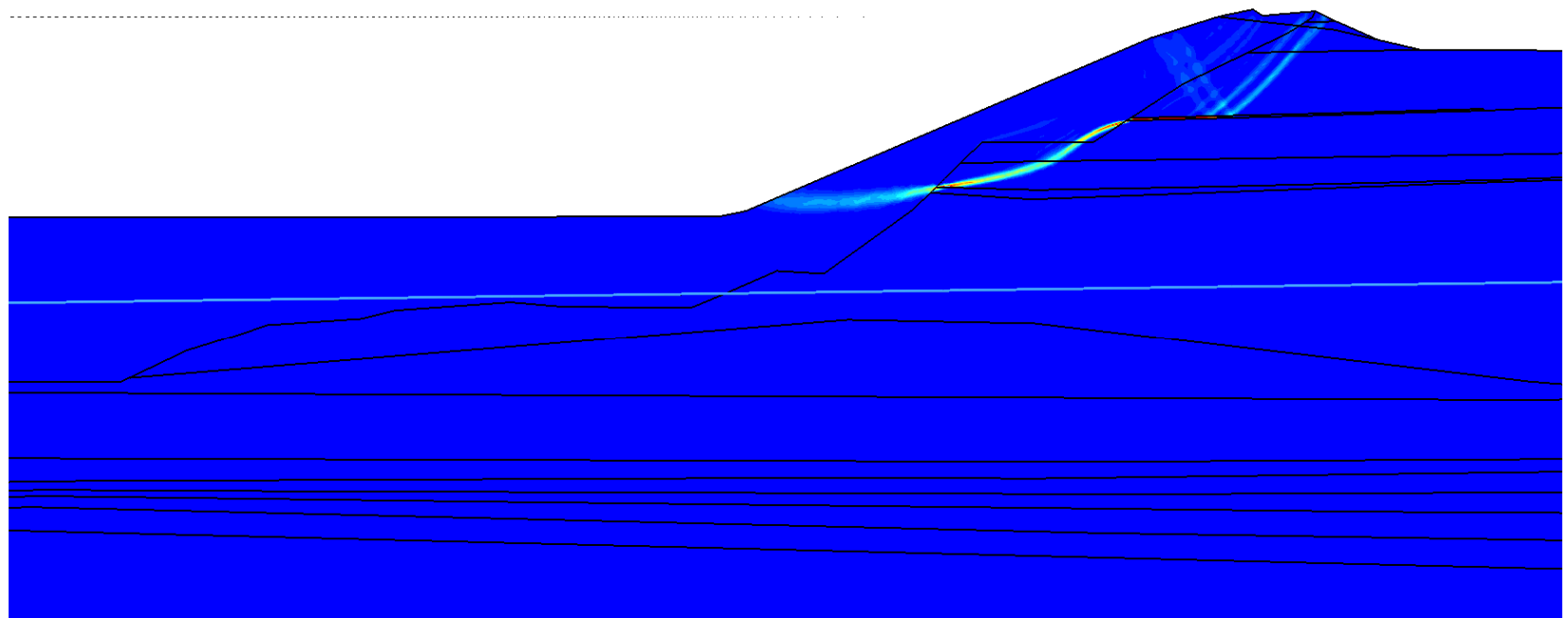
Abbildung 2: Potentieller Versagensmechanismus im prognostischen Zustand
