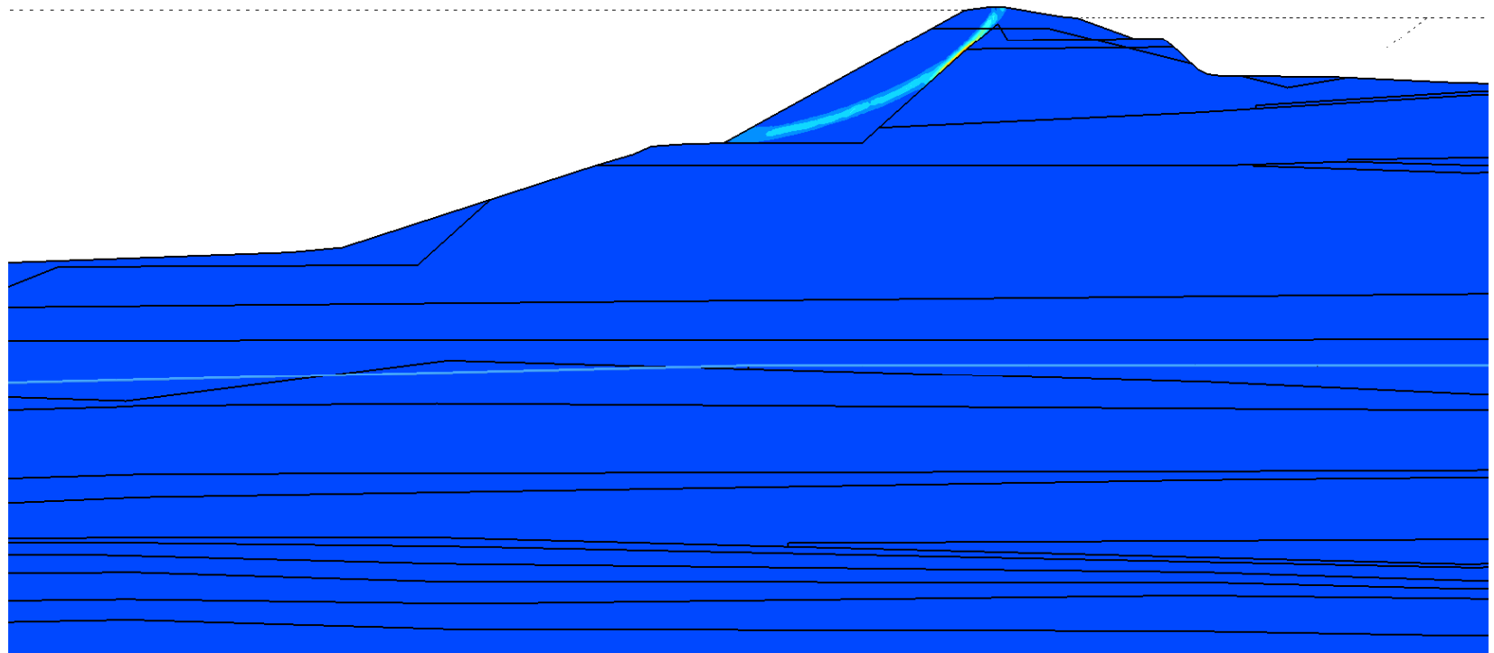
Abbildung 1: Potentieller Versagensmechanismus im aktuellen Zustand
