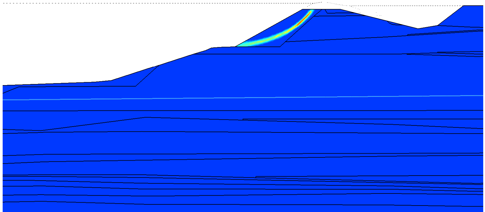
Abbildung 3: Potentieller Versagensmechanismus im prognostischen Zustand mit geplanten Maßnahmen aus Deponieerrichtung
