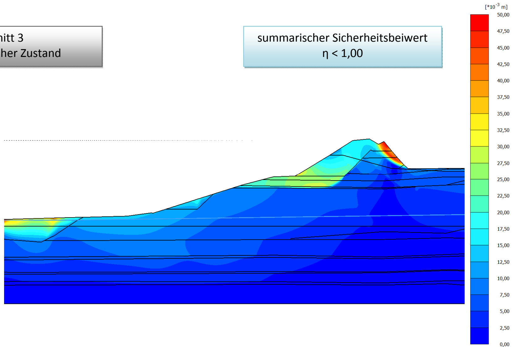
Abbildung 2: Inkrementelle Verschiebungen im prognostischen Zustand
