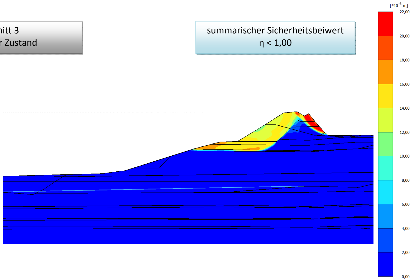
Abbildung 1: Inkrementelle Verschiebungen im aktuellen Zustand
