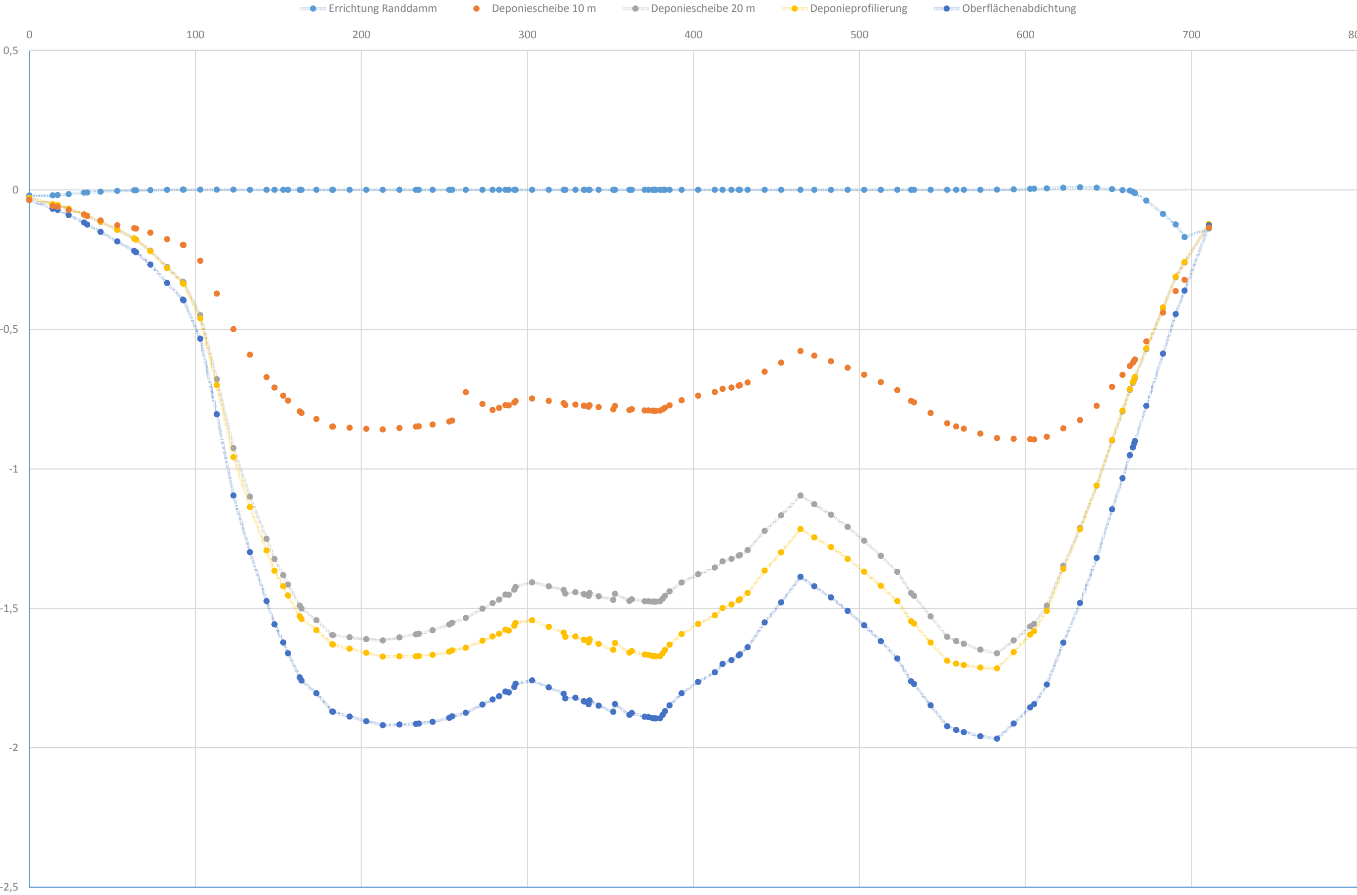
Schnitt 2 - Lastsetzungsverlauf - Berechnungsbasis Abschluss der Setzungen nach Herstellung der Basisabdichtung
