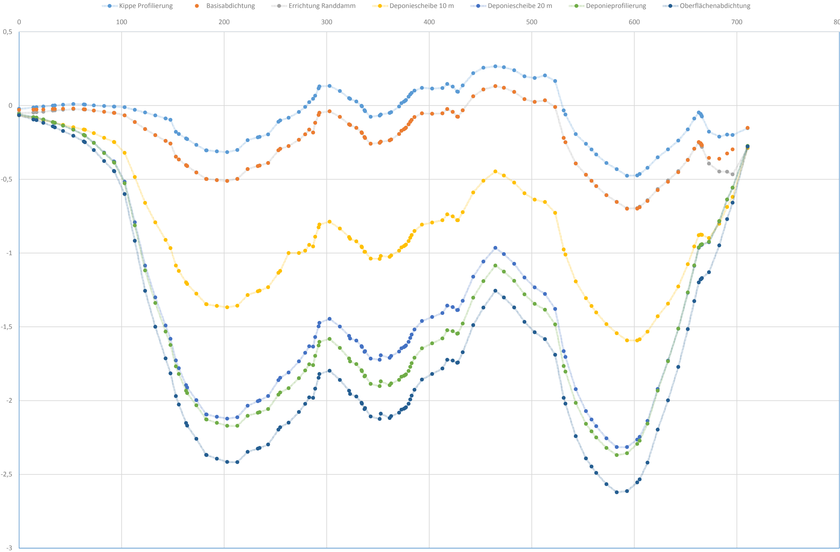
Schnitt 2 - Lastsetzungsverlauf - Berechnungsbasis InSitu-Zustand
