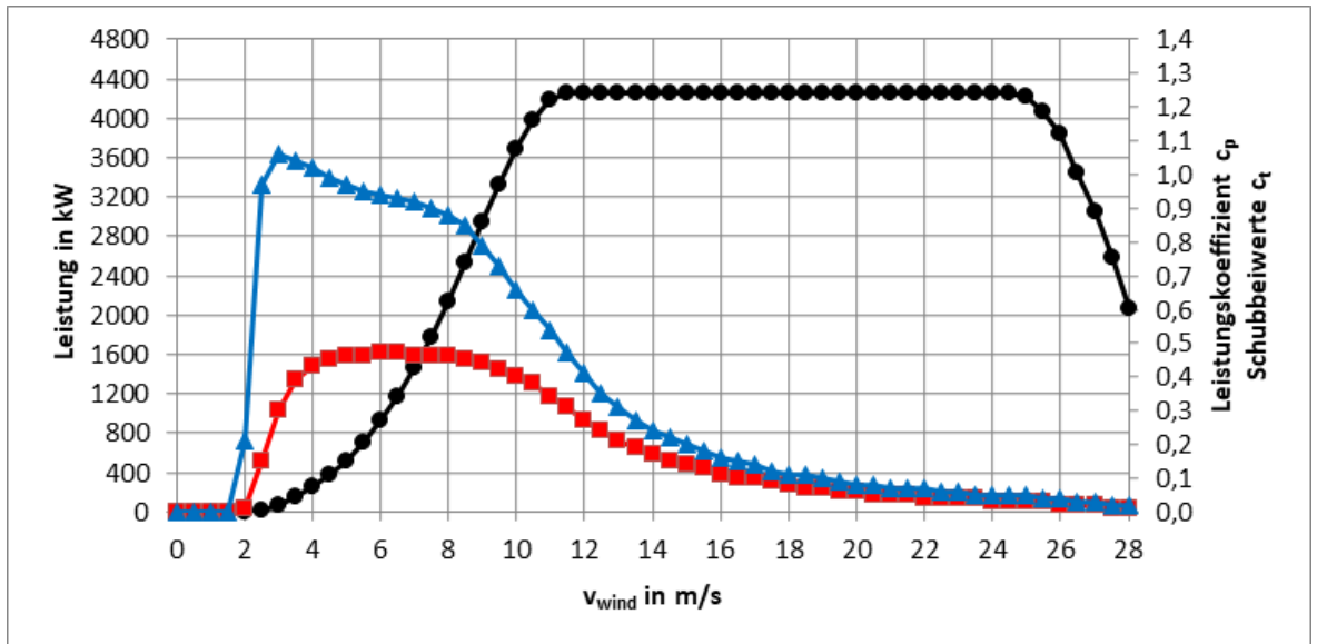
Abb. 1: Leistungs-, c_p - und c_t -Kennlinien E-138 EP3 E3 / 4260 kW Betriebsmodus OM-0-1
