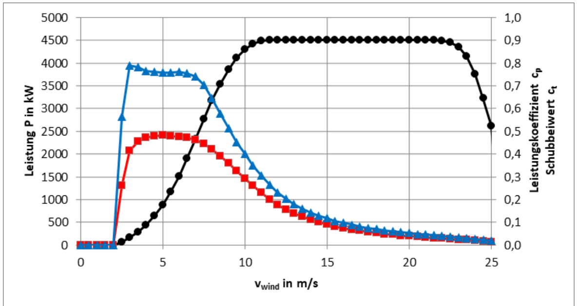
Abb. 1: Leistungs-, c_p - und c_t -Kennlinien E-175 EP5 E2 / 7000 kW Betriebsmodus OM-NR-03-0
