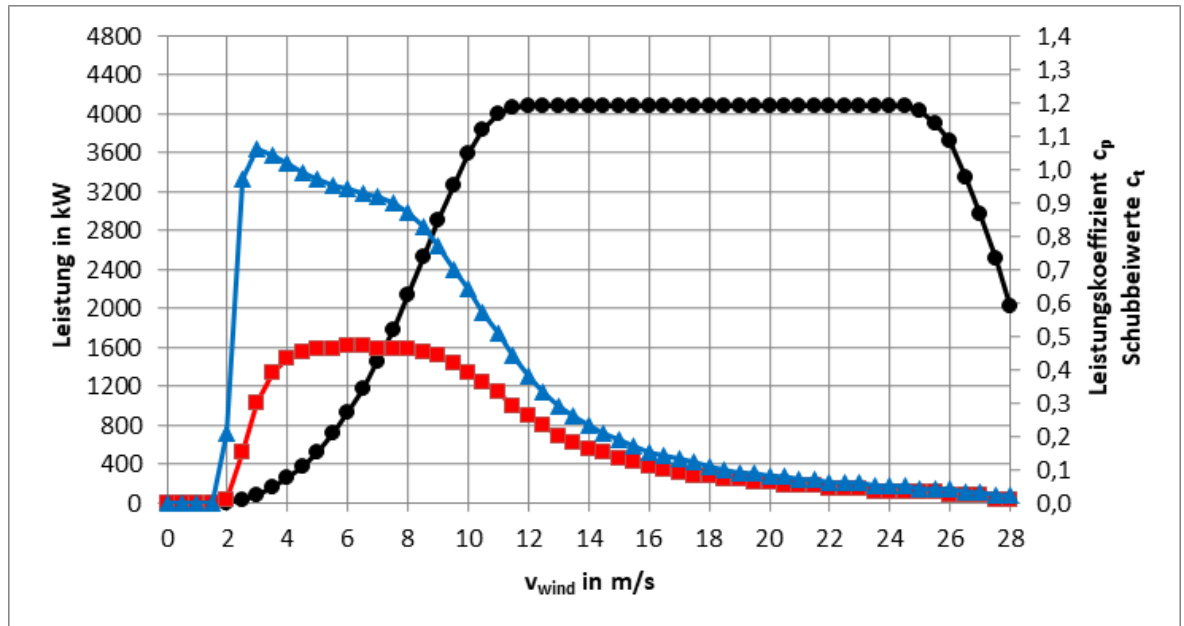
Abb. 1: Leistungs-, c_p - und c_t -Kennlinien E-138 EP3 E3 / 4260 kW Betriebsmodus OM-NR-01-1
