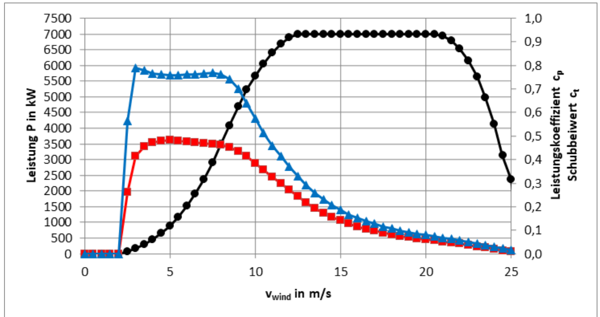
Abb. 1: Leistungs-, c_p - und c_t -Kennlinien E-175 EP5 E2 / 7000 kW Betriebsmodus OM-0-0
