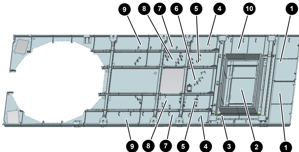
Abb. 12: Boden Maschinenhausverkleidung
