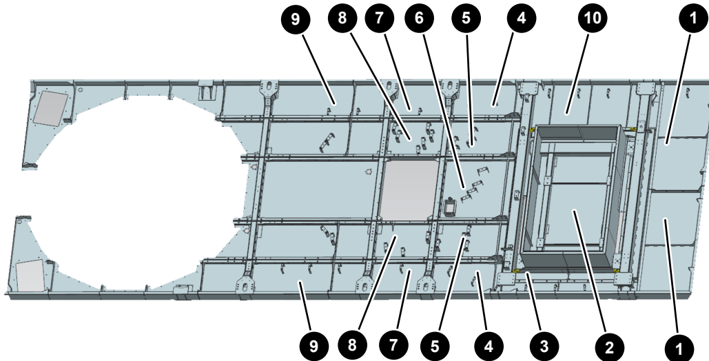
Abb. 8: Boden Maschinenhausverkleidung
