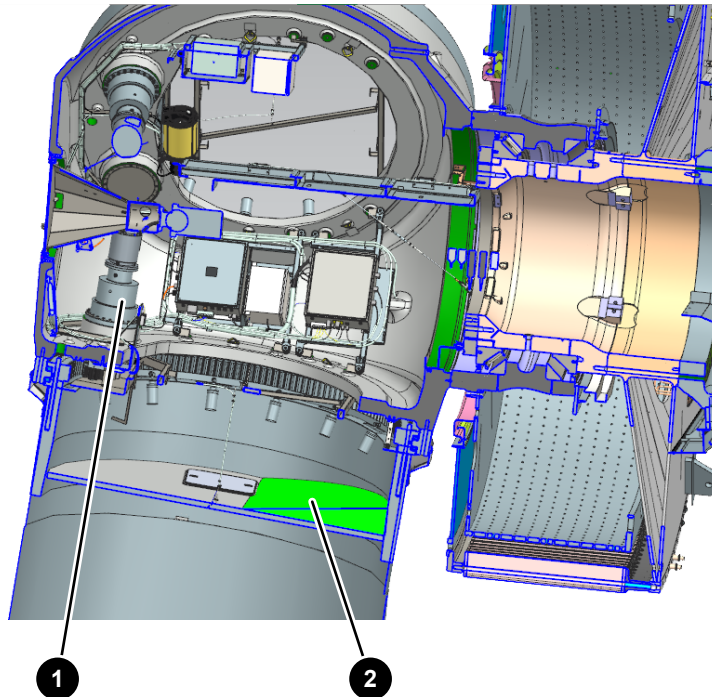
Abb. 4: Rotornabe mit Rotorblatt
