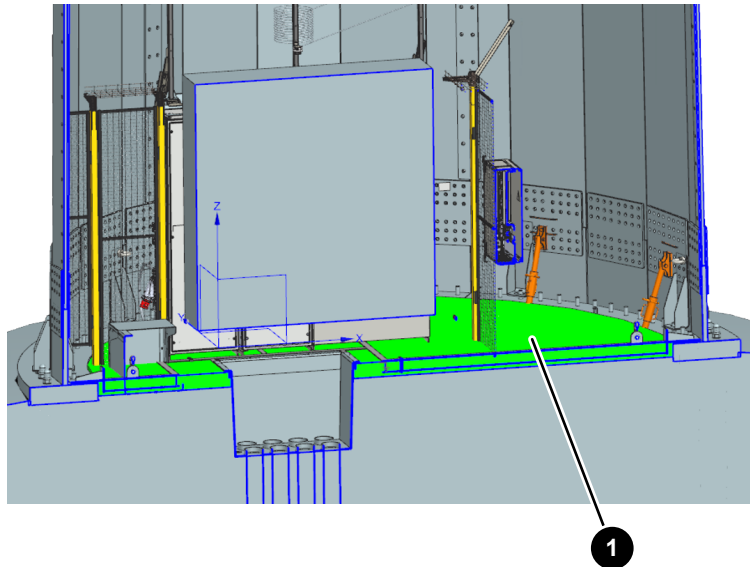
Abb. 7: Auffangmöglichkeit Turmboden
