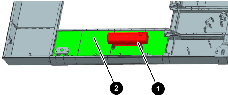
Abb. 11: Automatisches Löschesystem
