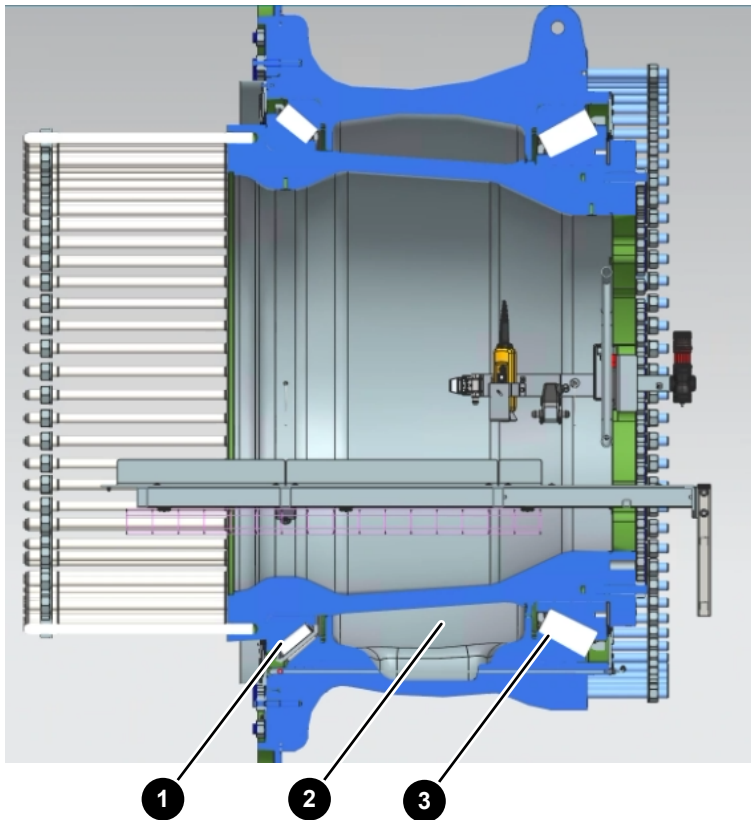
Abb. 6: Rotorlager
